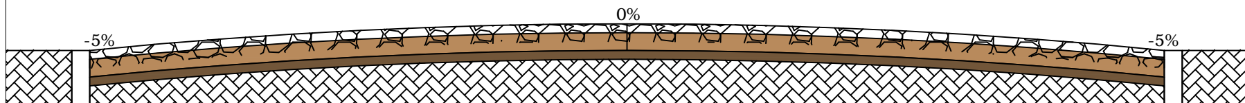
Corte Transversal do Calçamento
