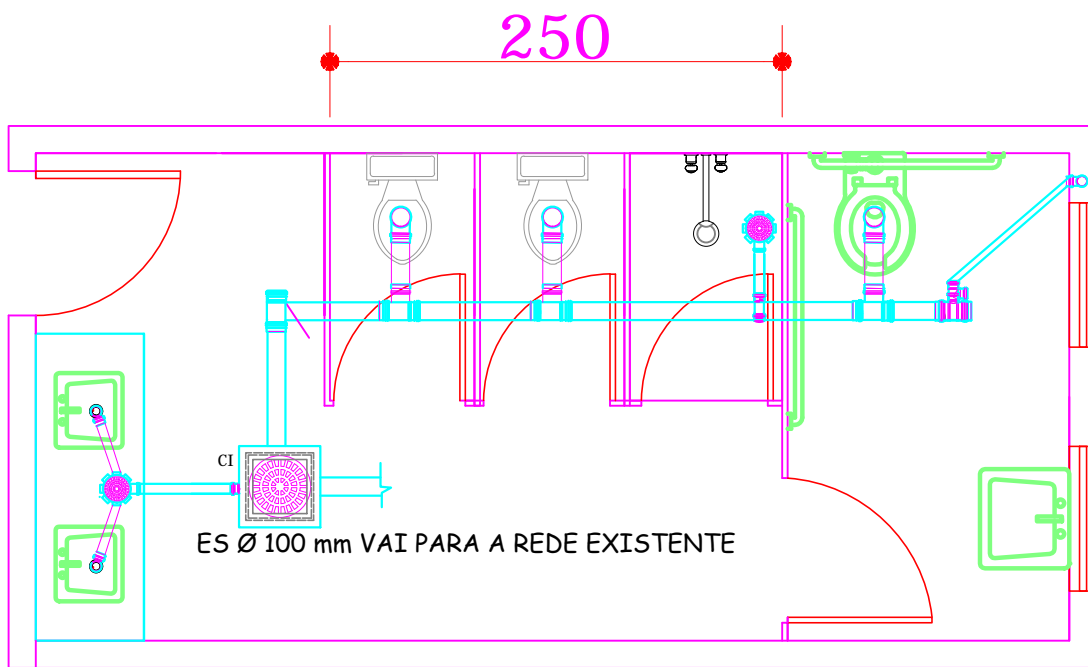
Instalação hidrossanitária
