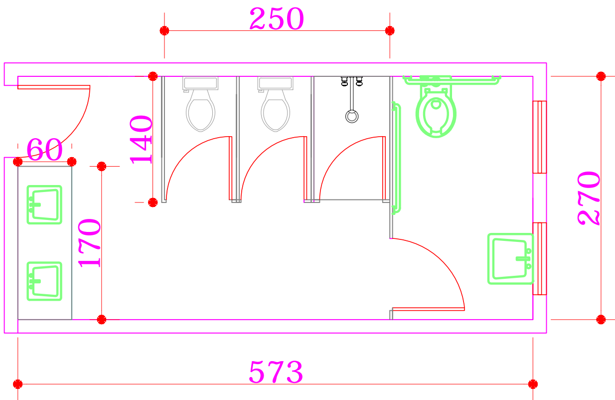
Planta baixa
